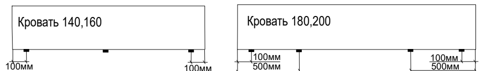
Схема установки подпятников
